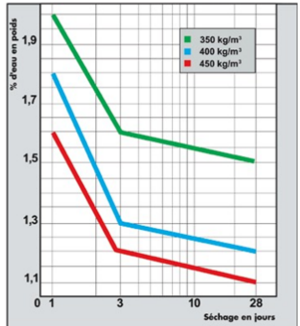
HUMIDITÉ RÉSIDUELLE DE LA CHAPE MAPECEM
