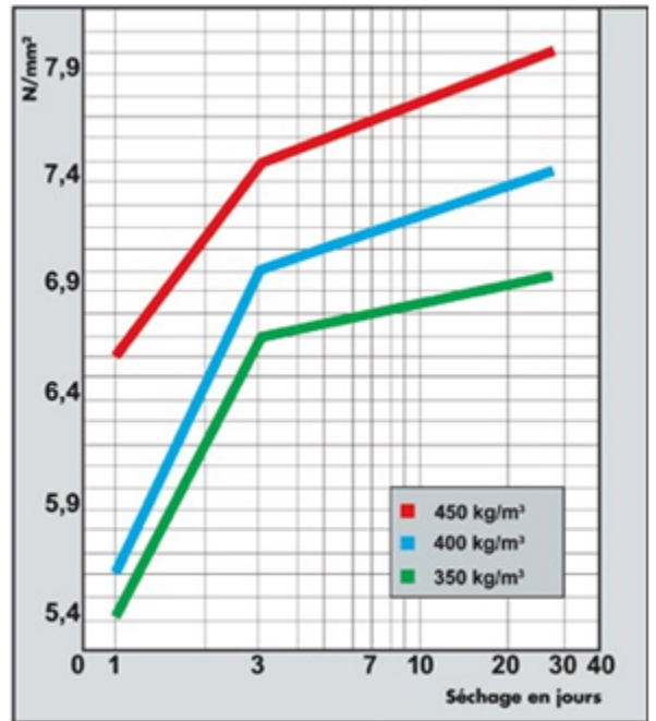
RÉSISTANCE À LA FLEXION DE MAPECEM À DIVERS DOSAGES
