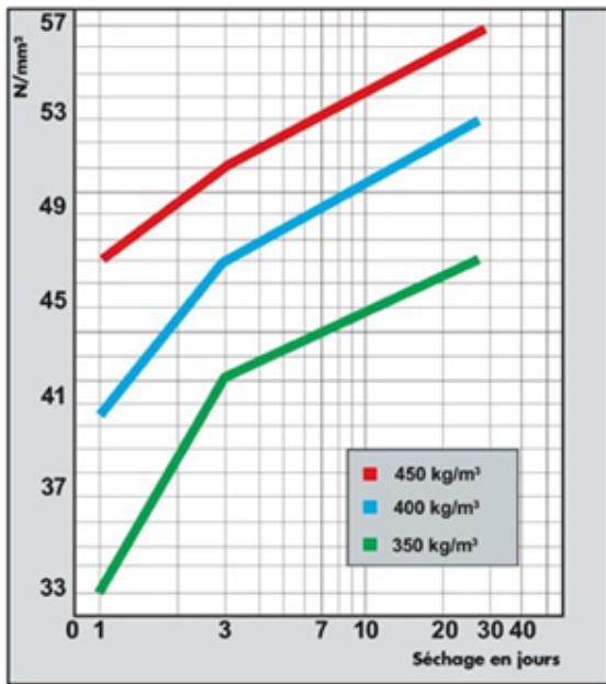
RÉSISTANCE À LA COMPRESSION DE MAPECEM À DIVERS DOSAGES
